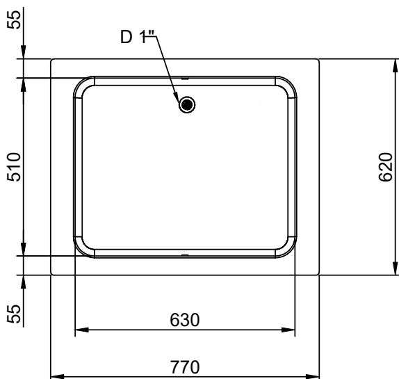
Päältä
